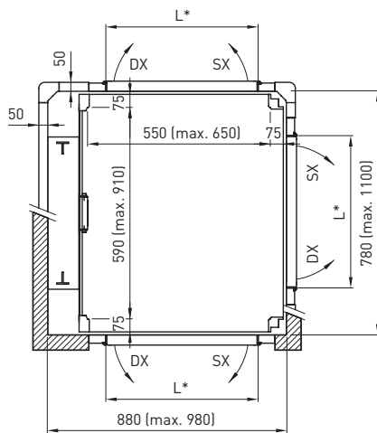
Cabin door side C
