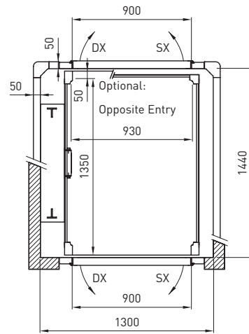
Cabin door side B
