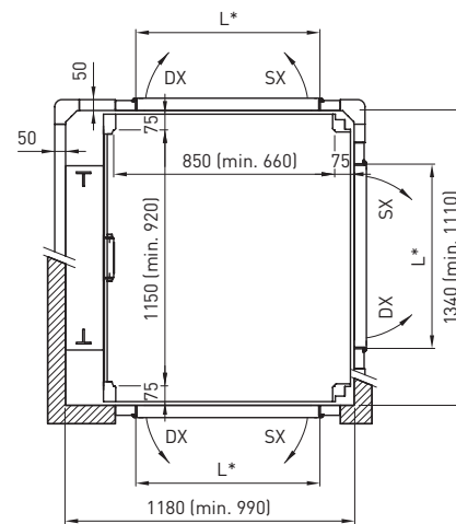
Cabin door side A,C
