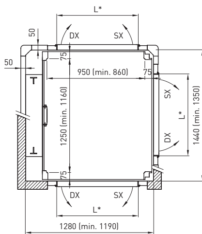
Cabin door side A,B
