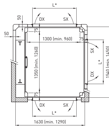
Cabin door side B,C
