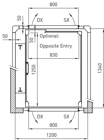
Cabin door side A
